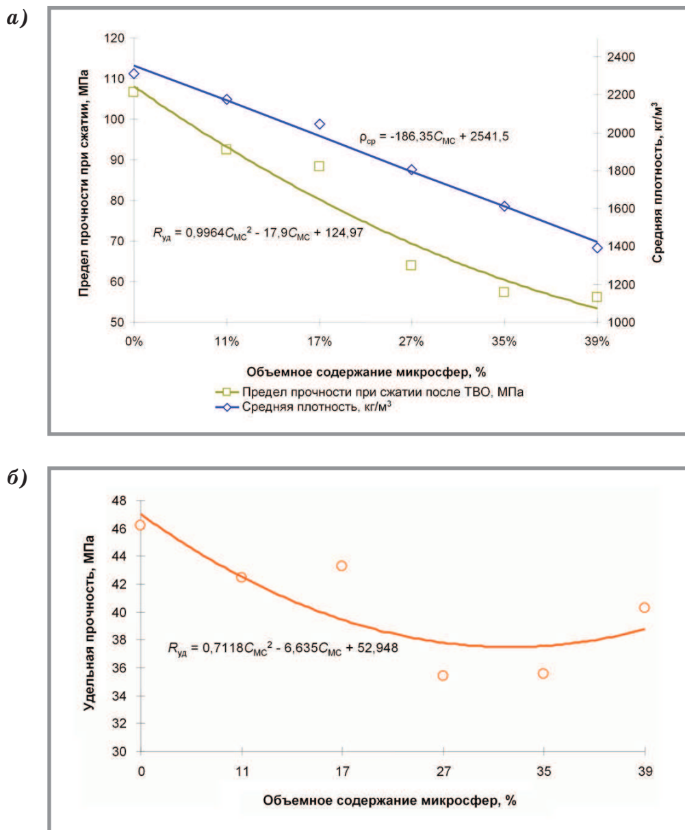
Рис. 2. Физико-механические свойства наномодифицированных высокопрочных легких бетонов: а – зависимость предела прочности при сжатии и средней плотности от содержания микросфер; б – зависимость удельной прочности от содержания микросфер
