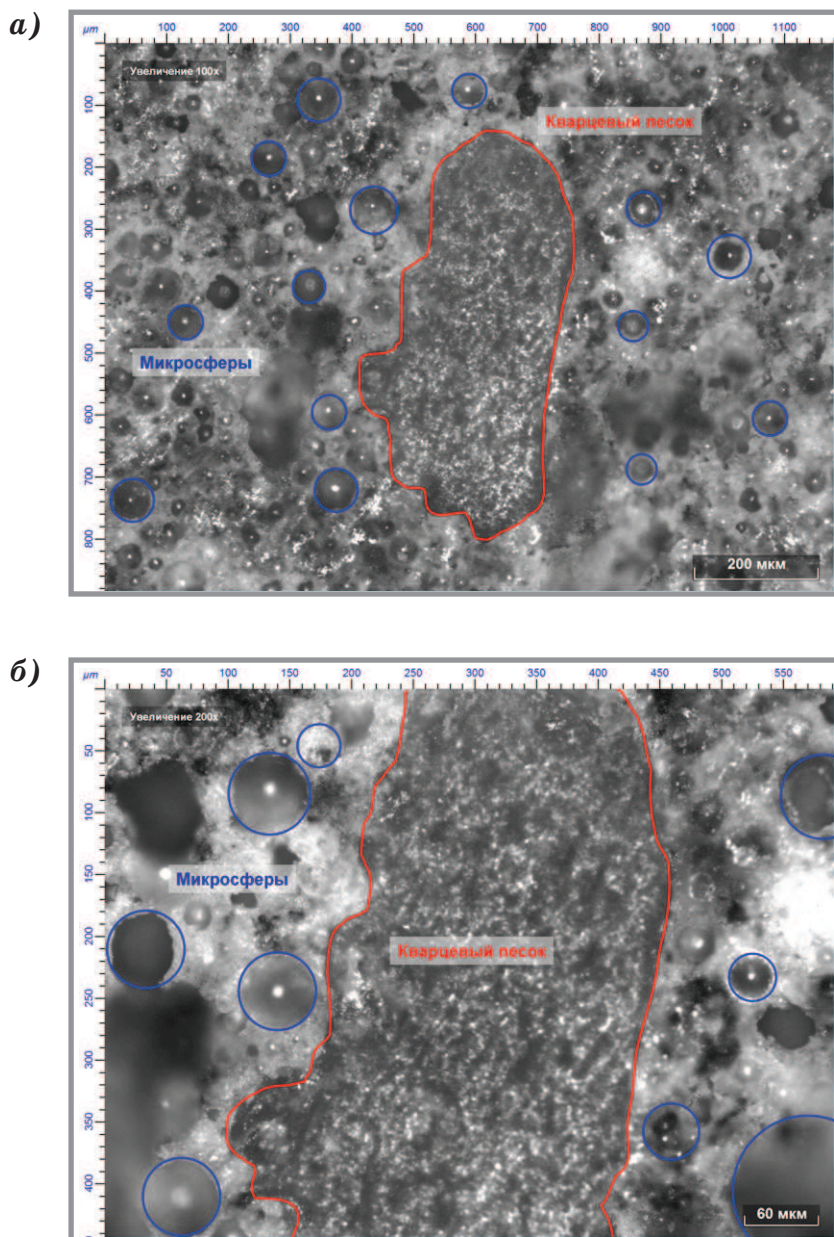
Рис. 4. Микрофотография структуры наномодифицированных высокопрочных легких бетонов: а – увеличение x100; б – увеличение x200
