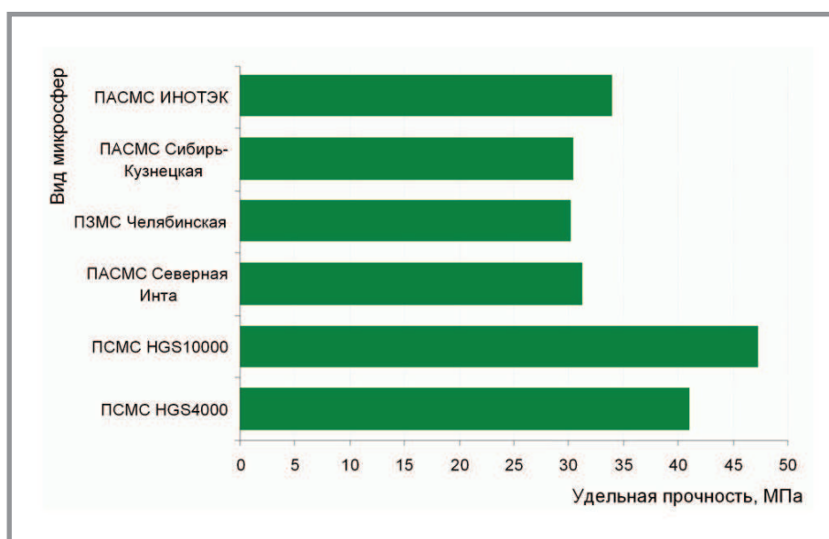
Рис. 1. Влияние вида микросфер на удельную прочность высокопрочных легких бетонов: ПСМС – полые стеклянные микросферы; ПАСМС – полые алюмосиликатные микросферы; ПЗМС – полые золомикросферы
